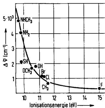
Abbild. 5 Verschiebung der längstwelligsten Bande ins Langwellige bei Benzolderivaten als Funktion der Ionisationsenergie (Elektronegativität)
