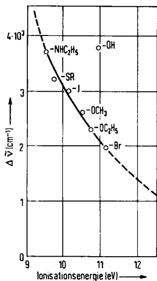
Abbild. 6 Verschiebung des Fluoreszenzmaximums bei Siloxenderivaten als Funktion der Ionisationsenergie (Elektronegativität)
